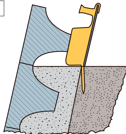
断面図
